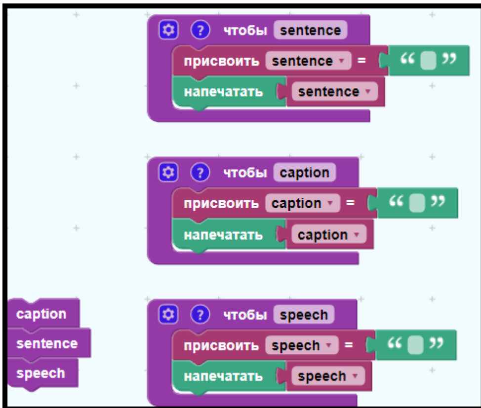
Рис. 5. Шаблон программы
